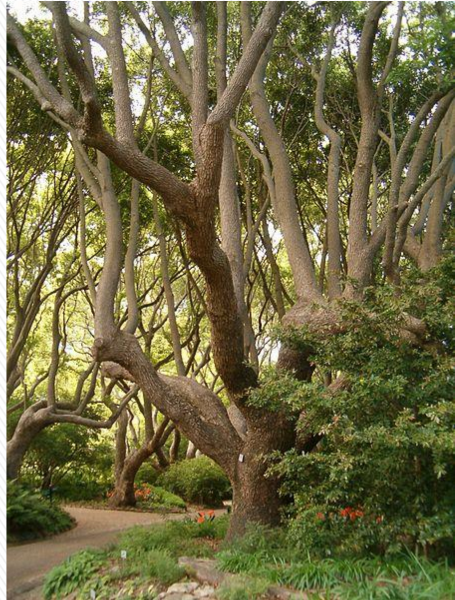
Obr. 45 skořicovník
