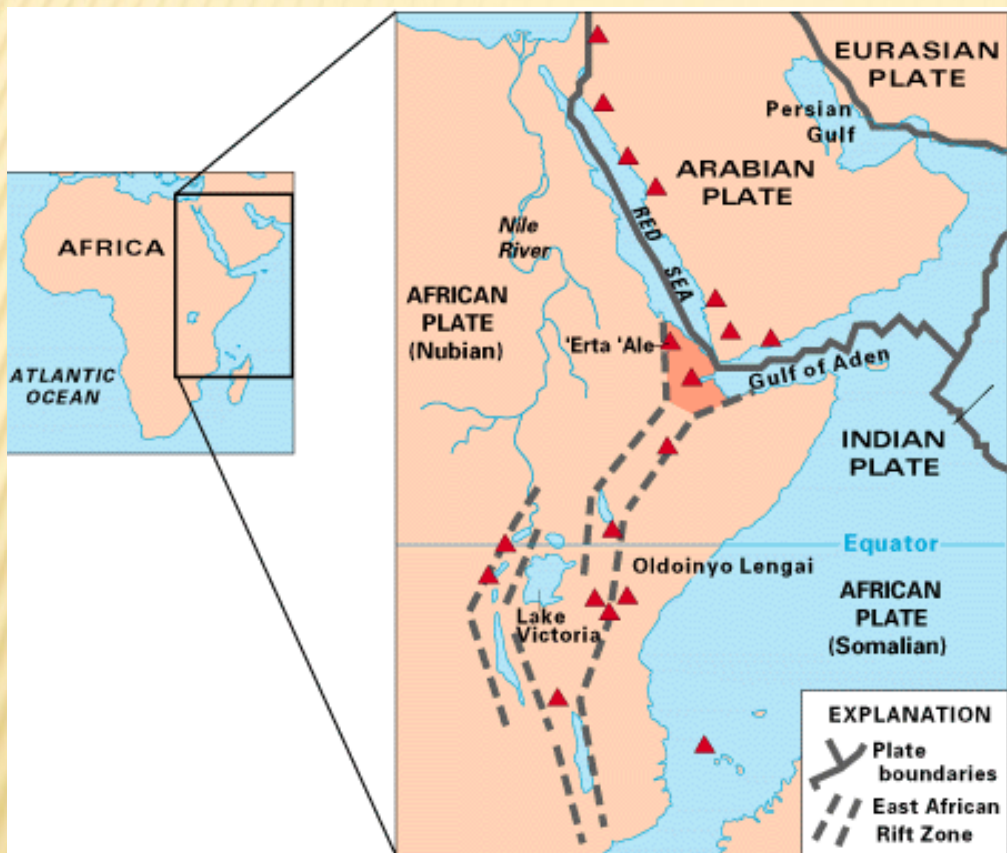
Obr. 5 Východoafrická příkopová propadlina
