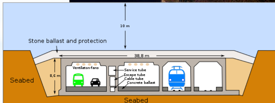
Obr. 36 Drogden tunel (3,5 km)
