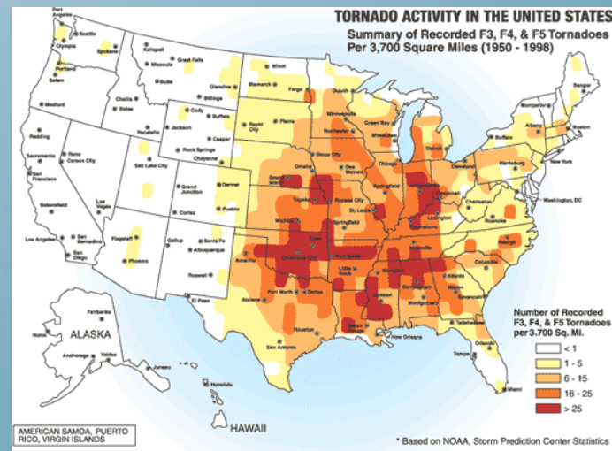
Obr. 15 Aktivita tornád v USA
