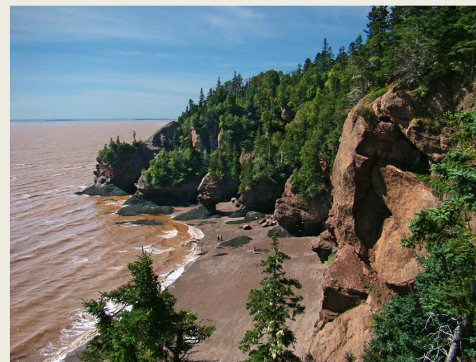
Obr. 7 Odliv, rozdíl hladin 17 m
